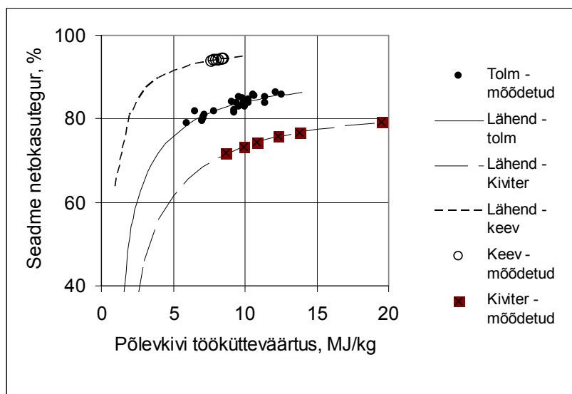
Pilt 4.3. Seosed põlevkivi utiliseerimisseadmete kasuteguri ja kasutatava põlevkivi kütteväärtuse vahel.
