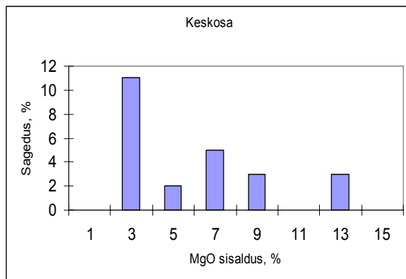
Pilt 7.2. Põlevkivikihi magneesiumisisaldus maardla keskosas, ammendatud Jõhvi, Sompa ja Tammiku kaeveväljadel
